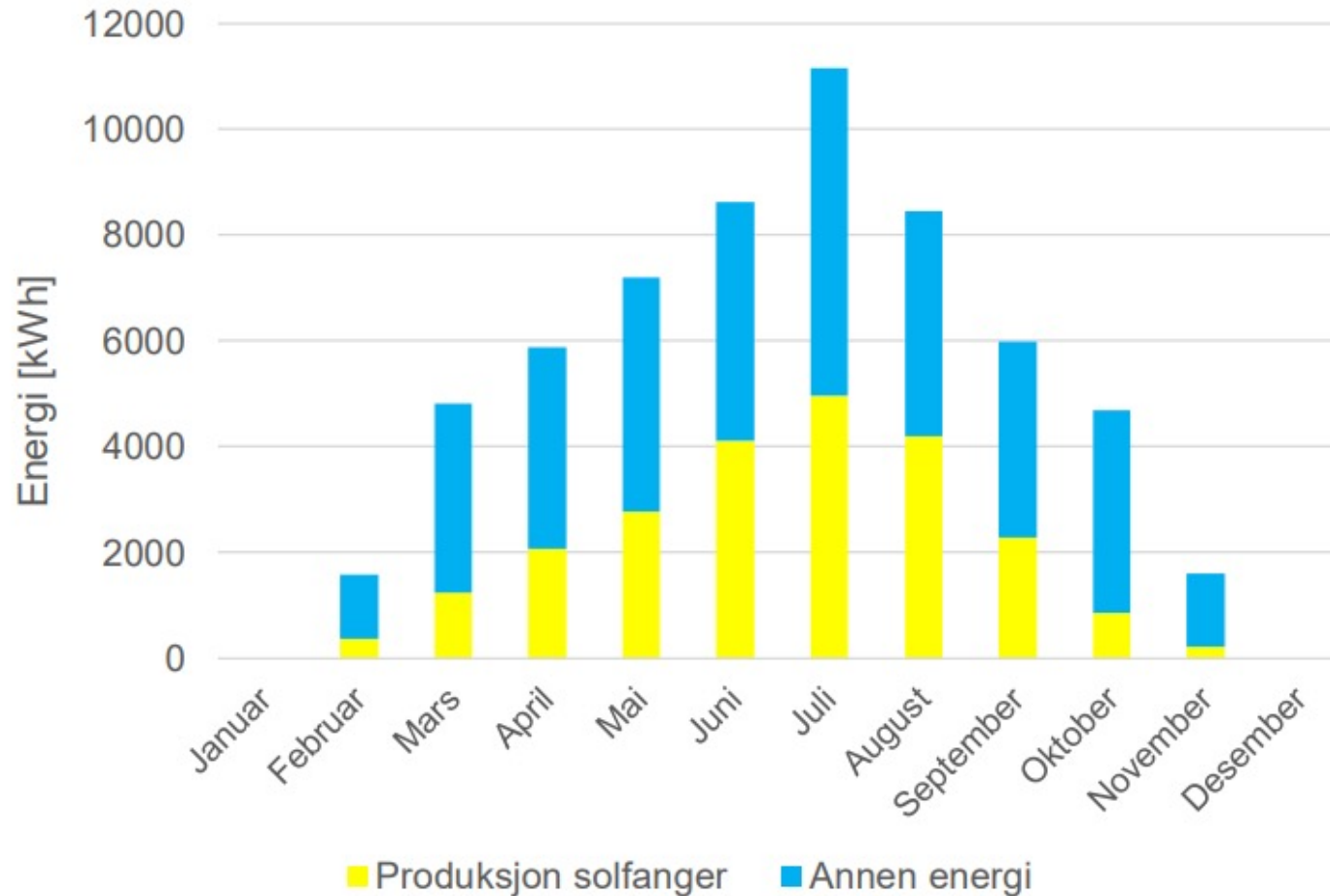
Figur 4: Varmeproduksjon fra 50 m 2 solfangere og nødvendig energimengde fra andre energikilder for å dekke totalt estimert oppvarmingsbehov av tappevann.
